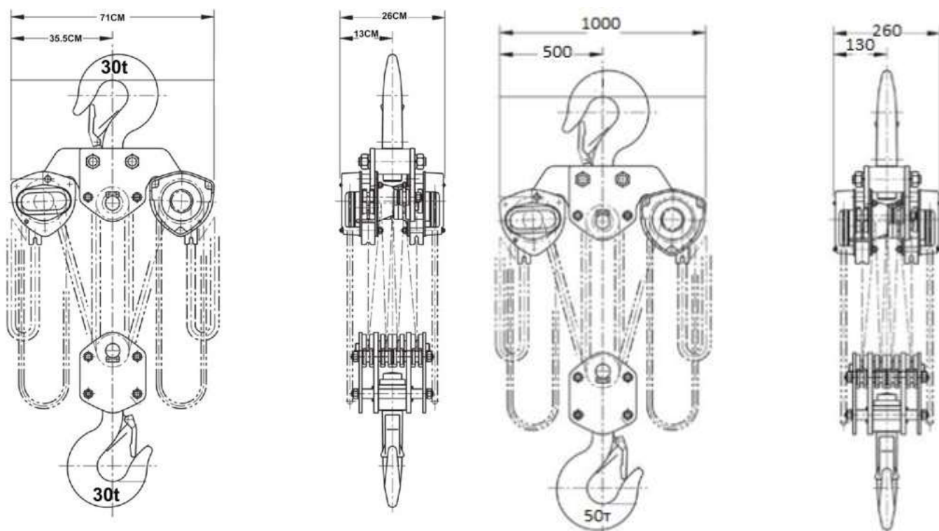
Грузоподъемность 30т Количество ветвей 12 Размер цепи 10X30
